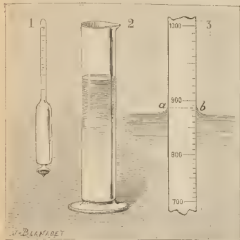
Fig. 1. Determinación de la densidad de un vino
